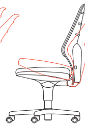
Regolazione dell'inclinazione del sedile bloccabile in multiposizione // Seat inclination adjustment lockable in multi position
